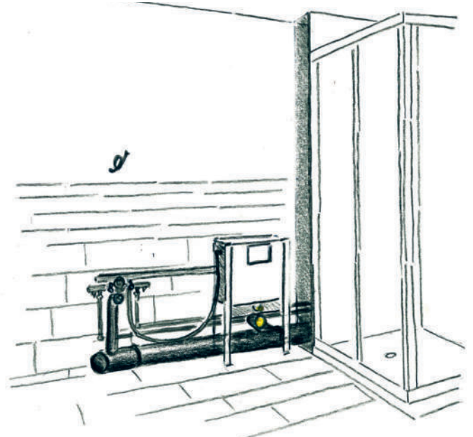
Version mit den Wasseranschlüssen am Sanitärrahmen Version avec raccords d'eau sur le cadre sanitaire
