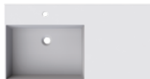
291 834 / 291 843 Lavabo Smart 50, 90 × 47 cm, coulée minérale K I Stone, sans trop-plein 291 834: avec tablette à gauche 291 843: avec tablette à droite
