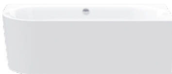
191 585 / 191 595 Baignoire Fresh Corner L, acryl, modèle d'angle avec tablier moulé, arrondi à gauche, garniture d'entrée, d'écoulement et de trop-plein chromée 191 595: XS, 155 × 80 × 60 cm 191 585: 180 × 80 × 60 cm
