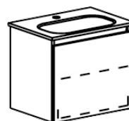
Unterbau ProCasa Tre 50 x 46 x 37,3 cm, für Keramikwaschtisch weiss, mit 1 Becken in der Mitte, Schubladenelement, 1 Schublade, mit Griffleiste, inkl. Raumsparisifon 954 205
