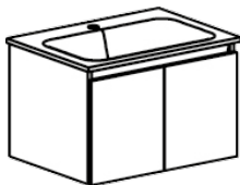
Unterbau ProCasa Tre 60 x 39 x 44,8 cm, für Keramikwaschtisch weiss, mit 1 Becken in der Mitte, 1 Unterbau 2 Türen, mit Griffleiste 954 201
